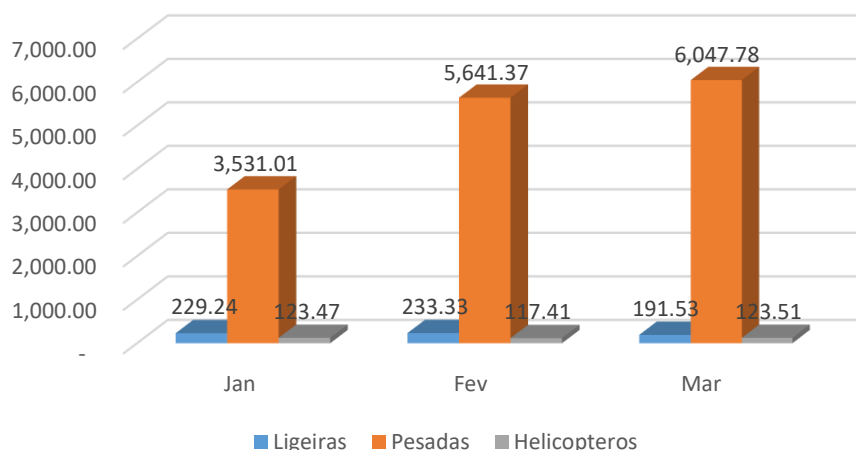
Emissões de CO 2 por Categoria de Aeronaves (TM)
